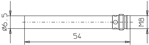
E2EL-C1R5□-M3L
