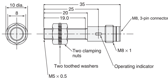
Fig. 36 : E2E-X1□□-M5
