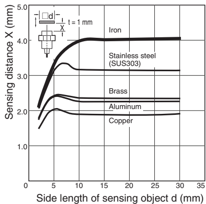
E2AX-M12□S04/ E2A-S12□S04
