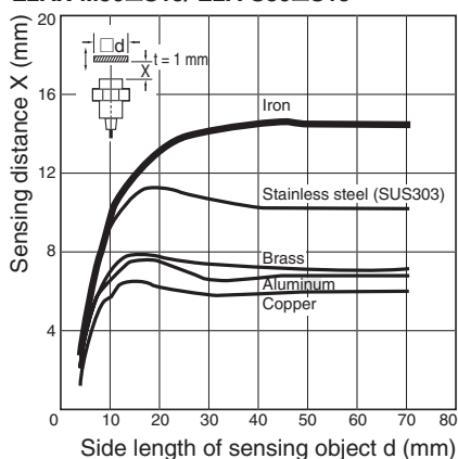
E2AX-M30□S15/ E2A-S30□S15
