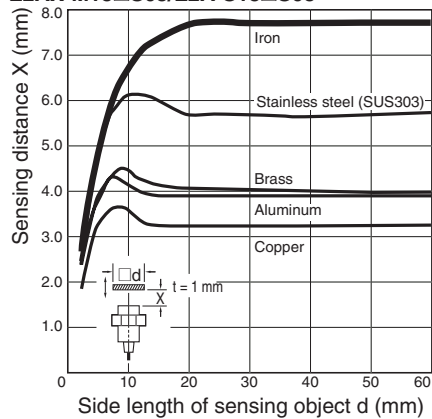
E2AX-M18□S08/E2A-S18□S08
