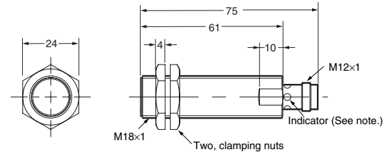
E2AU-M18LS08-M1-□□
